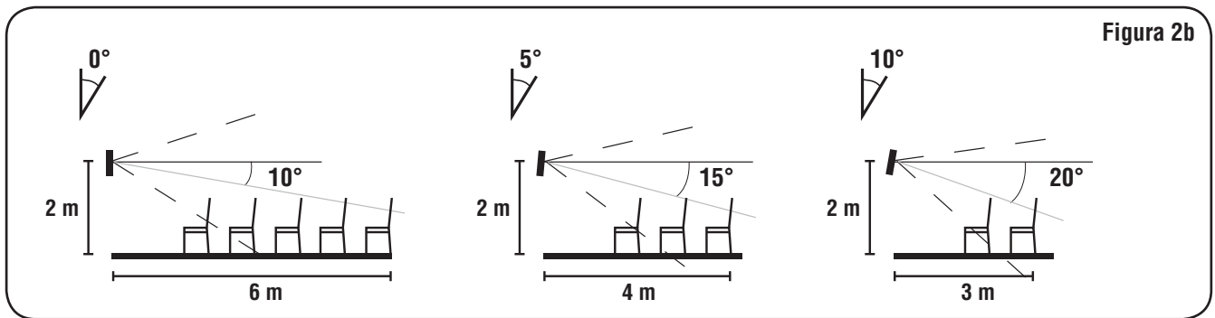
Figura 2b e 2c: esempi indicativi della copertura in funzione dell'angolo di inclinazione verticale della colonna sonora (installata in modo che il suo centro sia a 2 o 2,5 metri di altezza rispetto al pavimento).
